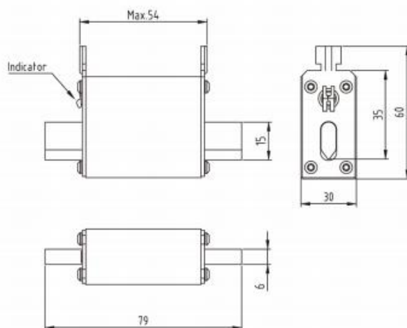
【Fig.-4G3A】 Unit: mm
