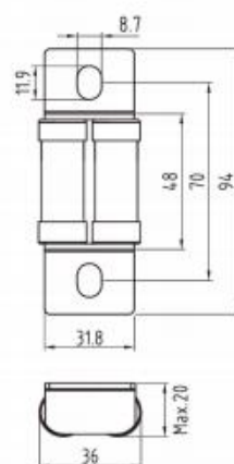
【Fig.-2F3A】 Unit: mm
