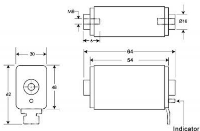
【Fig.4G4A】 Unit: mm
