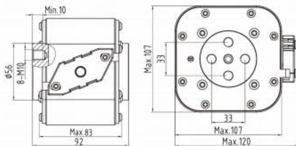
【Fig.-5G3A】 Unit: mm
