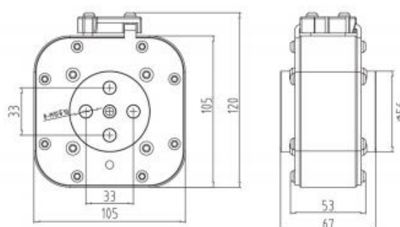
【图-5G2A】 Unit: mm
