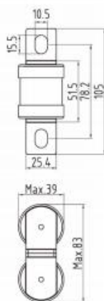
【Fig.-2F5A】 Unit: mm
