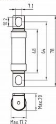
【Fig.-2F1A】 Unit: mm
