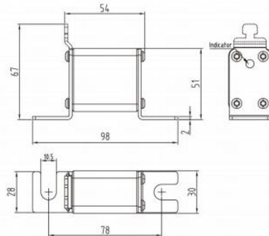
【Fig.-5G4A】 Unit: mm
