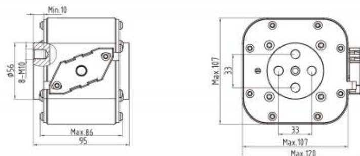
【Fig.-6G5A】 Unit: mm
