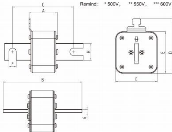
【Fig.-2G1A】 Unit: mm
