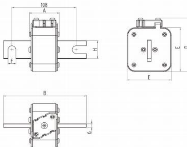
【Fig.-7G2A】 Unit: mm
