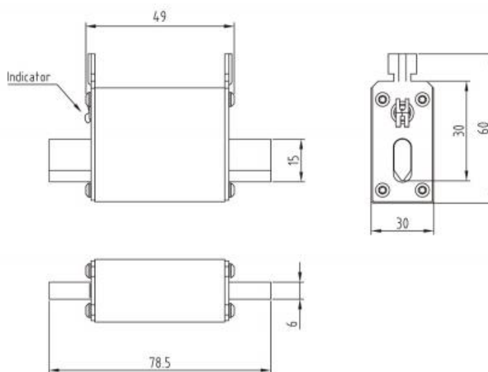
【Fig-6G3A】 Unit: mm
