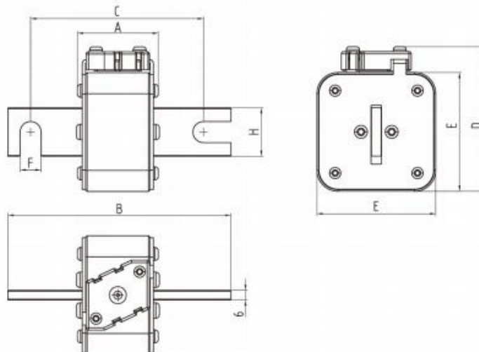
【Fig.-3G1A】 Unit: mm
