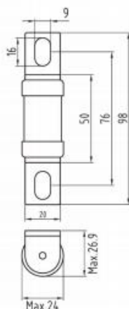
【Fig.-2F2A】 Unit: mm
